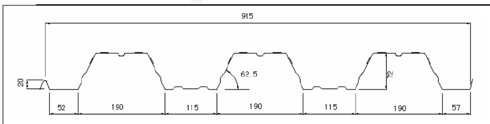
Plano producto acabado. Con nuestra visita se detectó errores. El plano indica 52 mm pero en realidad es 57 mm.
